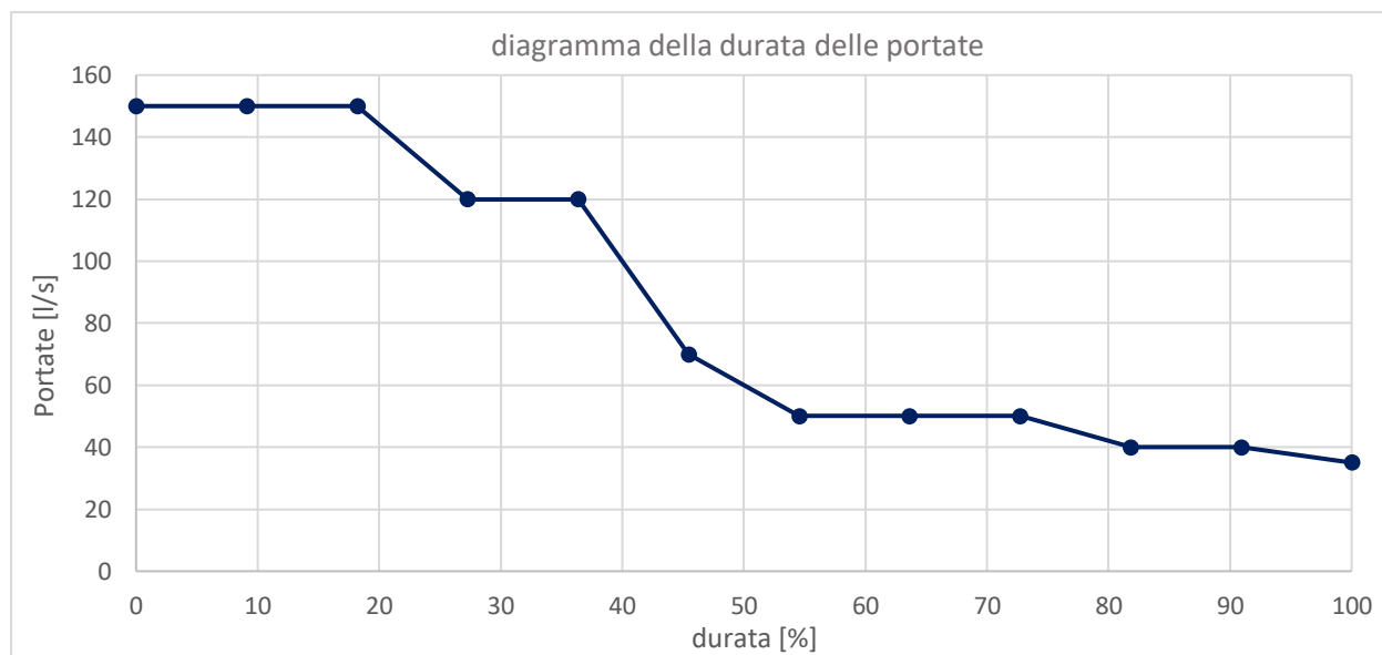
Figura 11.1: diagramma della durata delle portate
